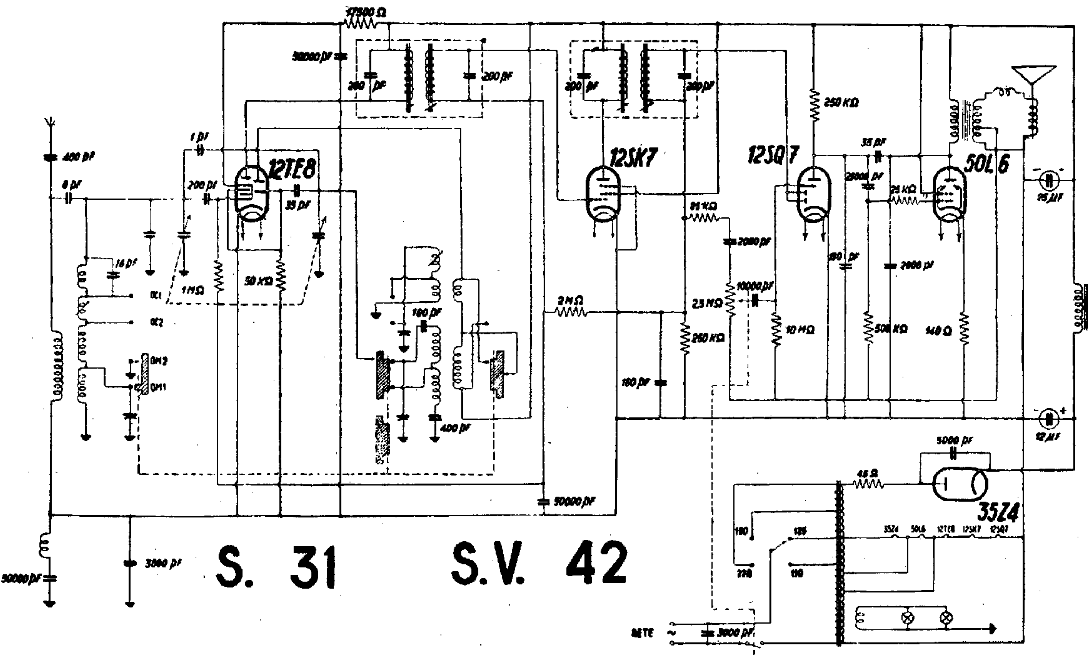
MAGNADYNE RADIO - Modelli SV 31 e SV 42 - Gamma onde medie divisa e due gamme onde corte. Media frequenza 471,5 kc/s. RN dalla placca della 50L6 con condensatore di 35 pF, e dal secondario trasformatore d'uscita. Potenza d'uscita 2 W. Filamenti in serie. 45 W circa di consumo.
